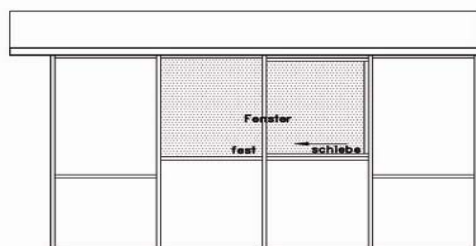
SEITENANSICHT RECHTS
